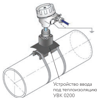
Измерение температуры трубы \varnothing \geq 57 мм
