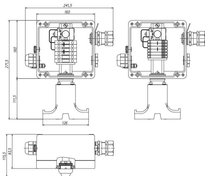
Коробка с винтовым (слева) и пружинным (справа) клеммным блоком
