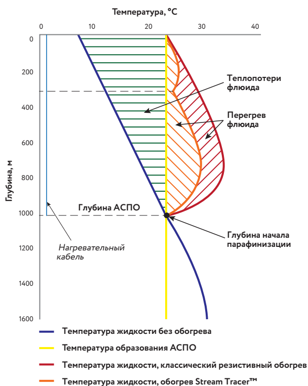
Энергоэффективность использования системы Stream Tracer™ по сравнению с резистивным кабелем
