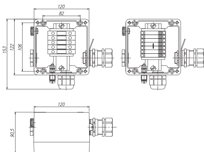
Коробка с винтовым (слева) и пружинным (справа) клеммным блоком
