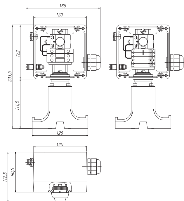
Коробка с винтовым (слева) и пружинным (справа) клеммным блоком
