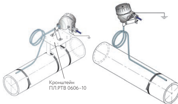
Измерение температуры трубы любого диаметра
